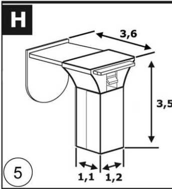
KRUVIVABA KINNITUS AB41 MUDELILE
