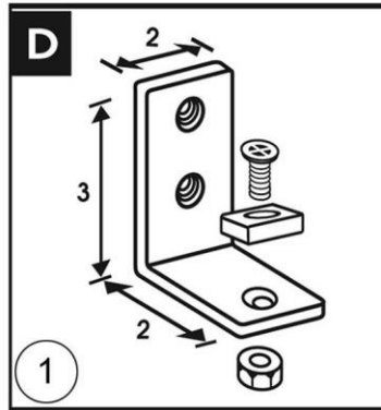
SEINAKINNITUS AB SÜSTEEMILE
