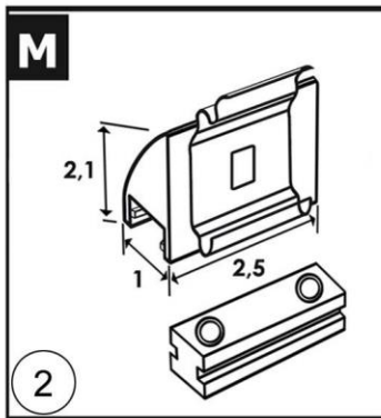
KLAASILIISTU KINNITUS PLASTIKUST LAEKINNITUSELE
