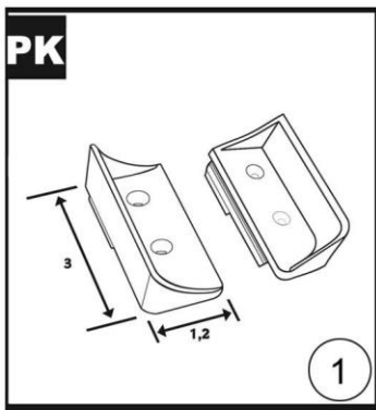
TALLAD KALDENURGA REGULEERIMISEKS KINNITUSELE "P"
