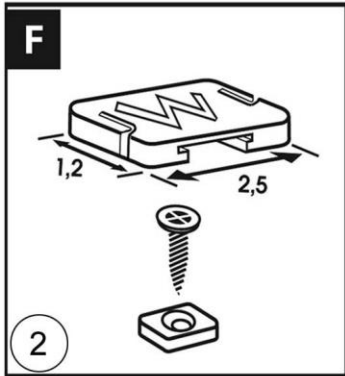
NÖÖRIKINNITUS (Standard AB süsteemil)
