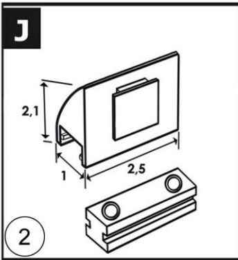
KLAASILIISTU KINNITUS PLASTIKUST AB SÜSTEEMILE
